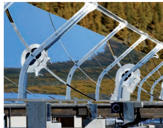
En plein été, les capteurs cylindro-paraboliques de Saignelégier couvrent jusqu'à 50% de l'énergie thermique consommée. © Photo : Agence Solaire Suisse
