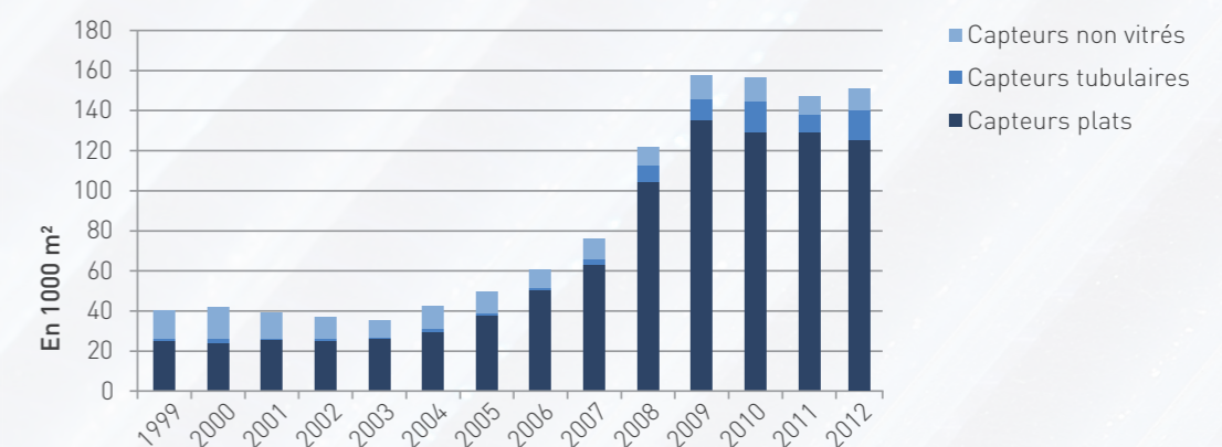
Surface de capteurs installée par an en Suisse
